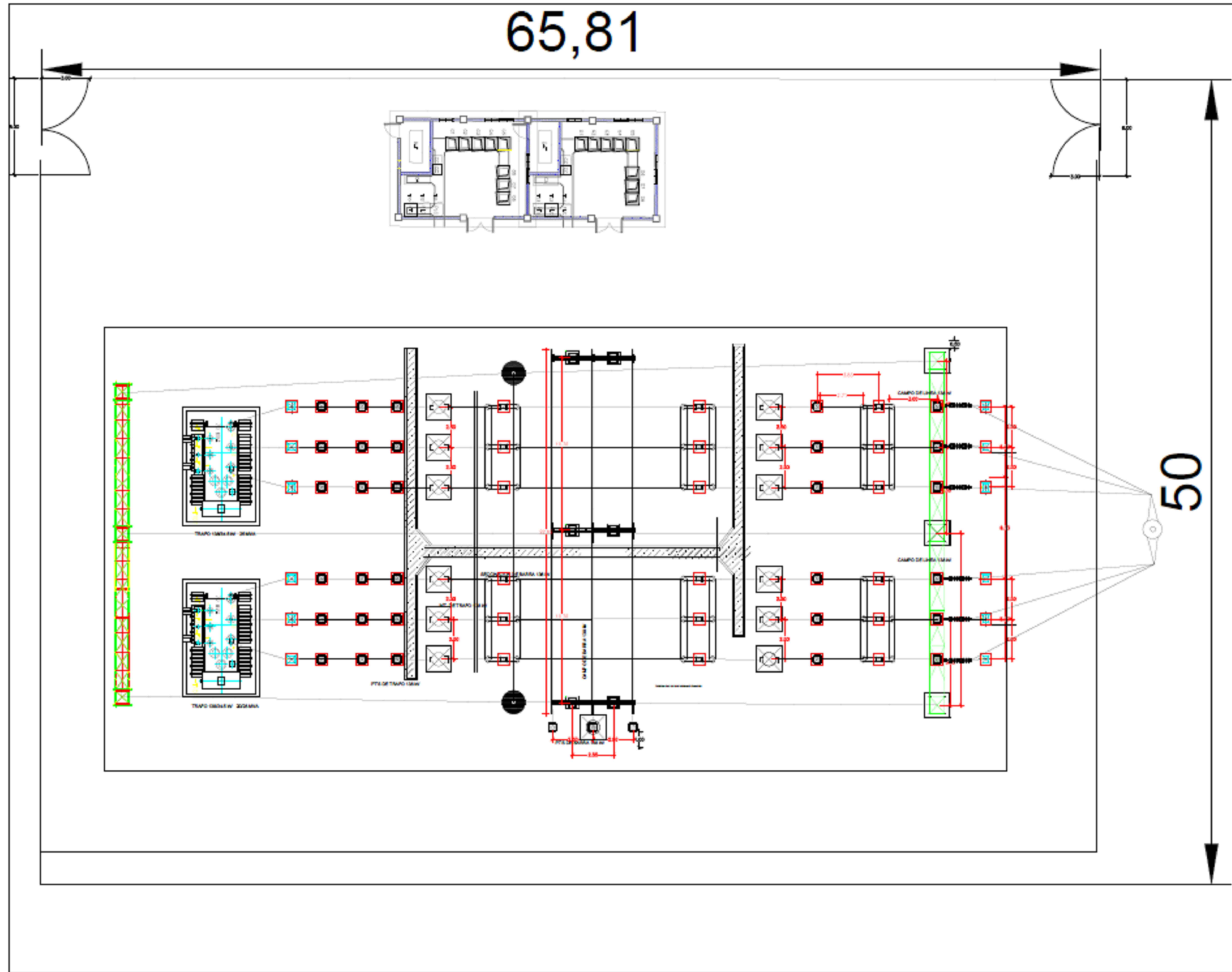
LAYOUT SUBESTACION 2X28MVA 138/34.5kV
