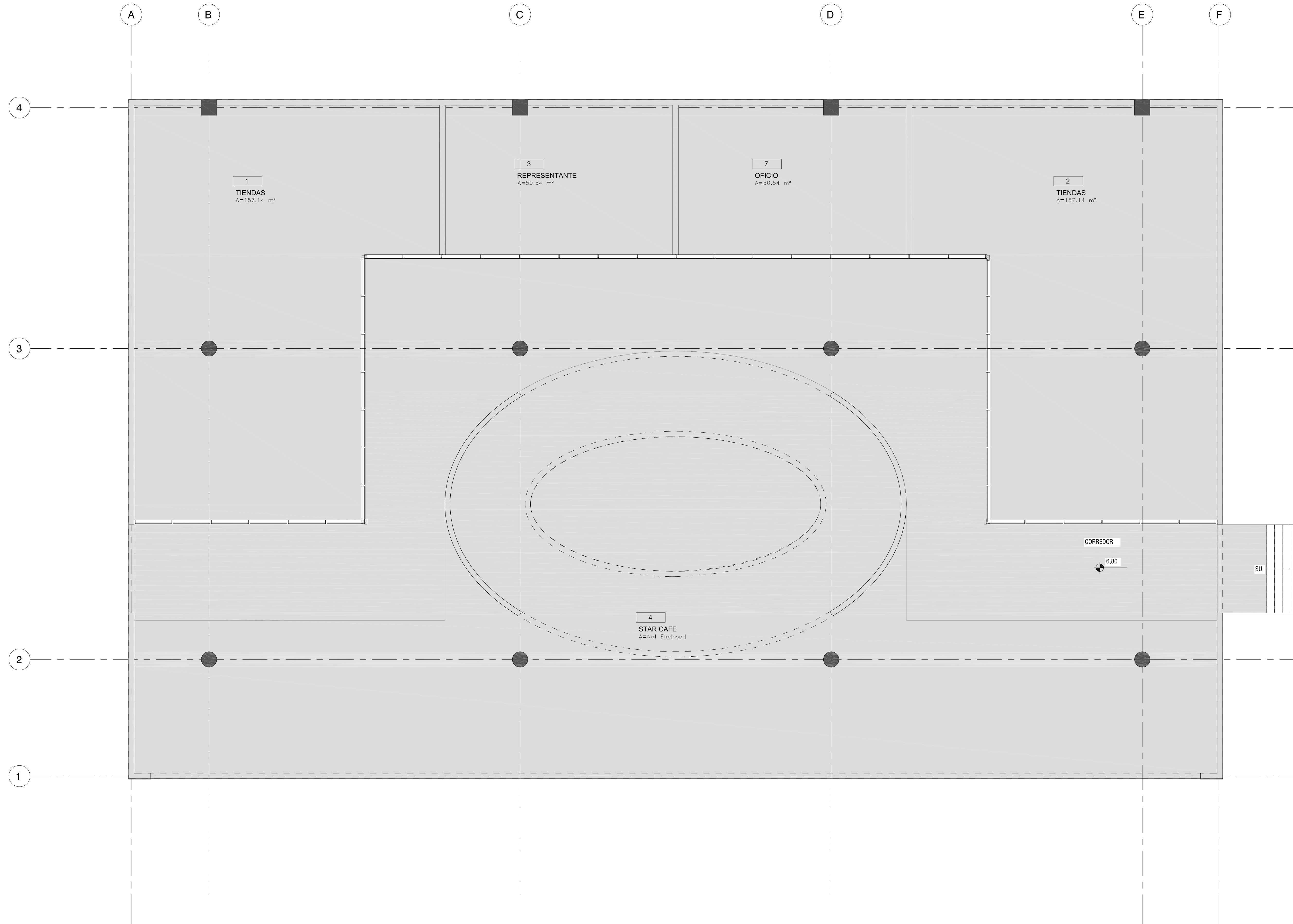
1 PLANTA ARQUITECTONICA 1ER NIVEL 1:75
