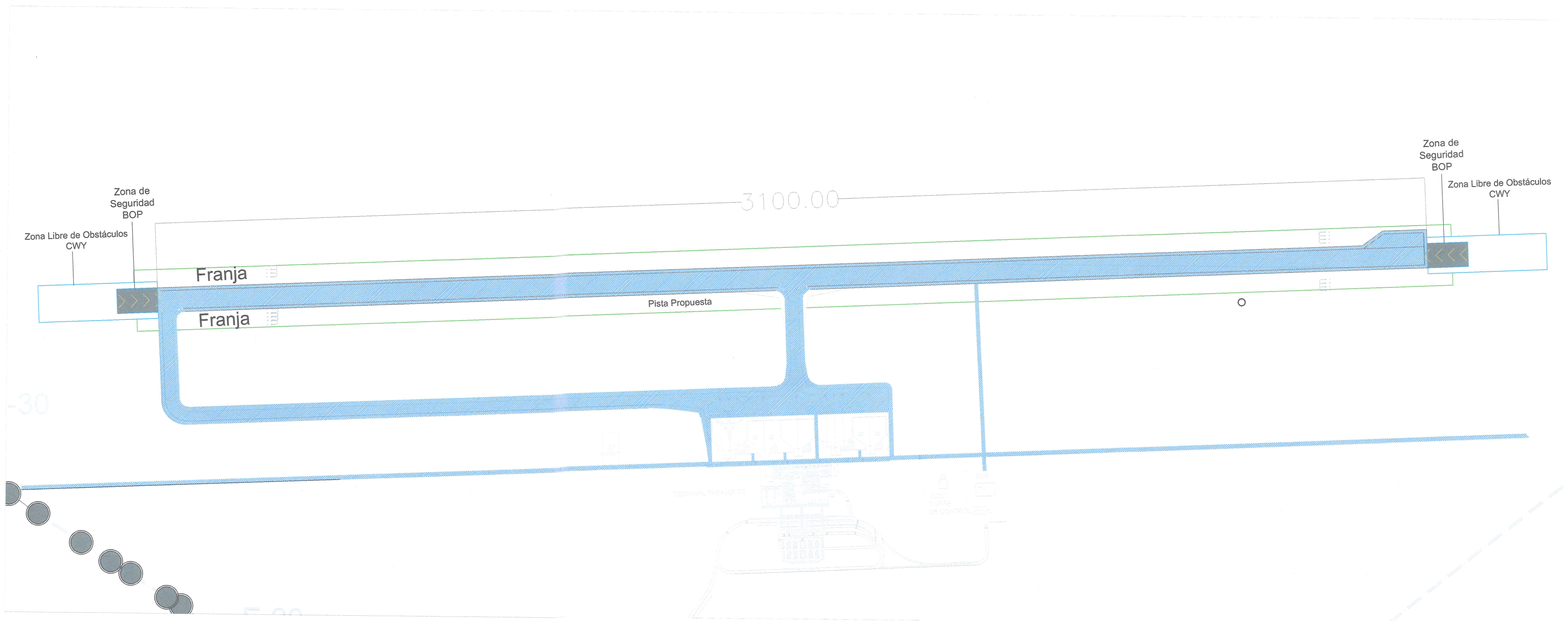
Planta composición de pavimento Pista de Vuelo
